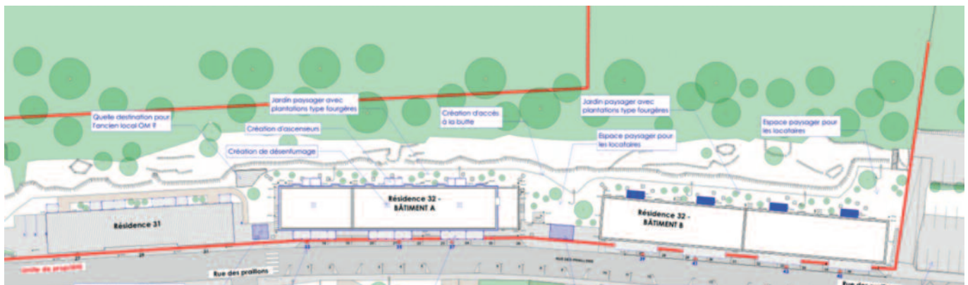
Figure 2 : Plan masse Phase DIAG site PRAILLONS
